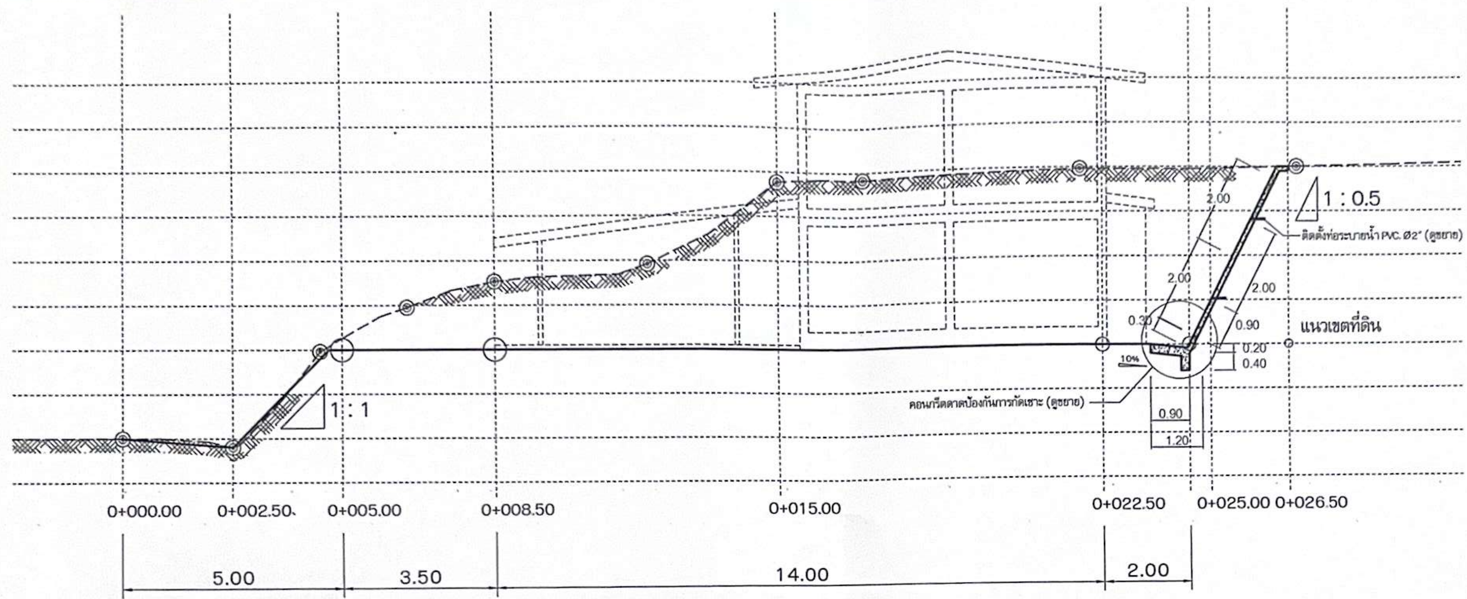
แบบแสดงคอนกรีตตาด ป้องกันการกัดเซาะ มาตรฐาน 1 : 100
